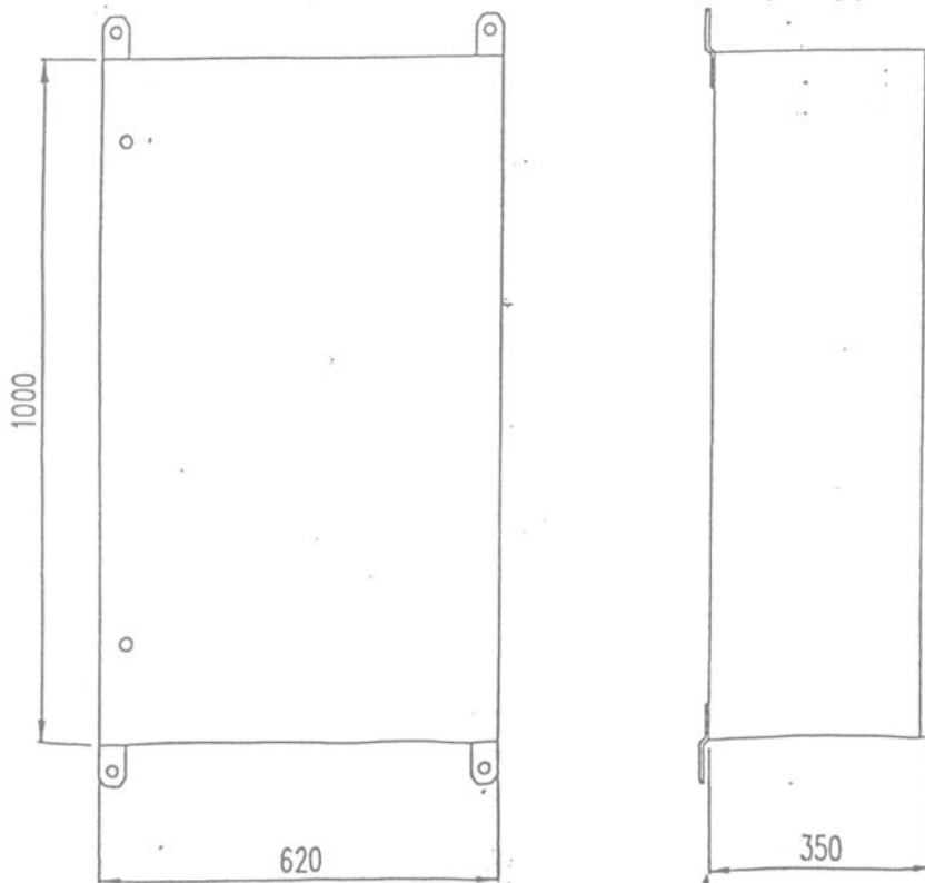
Шкаф управления
