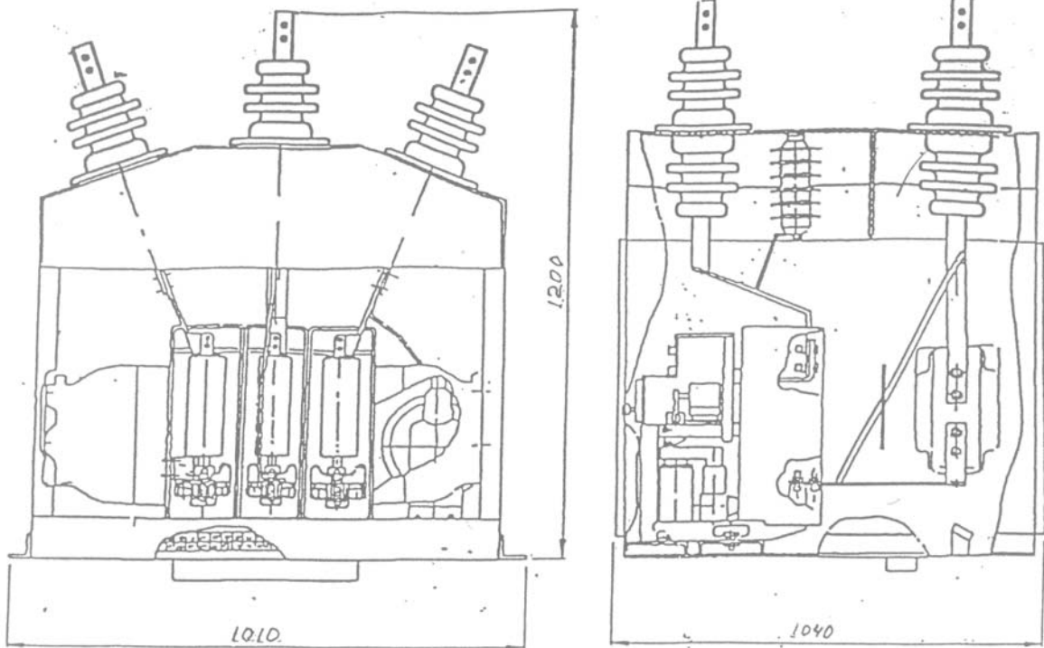
Шкаф управления
