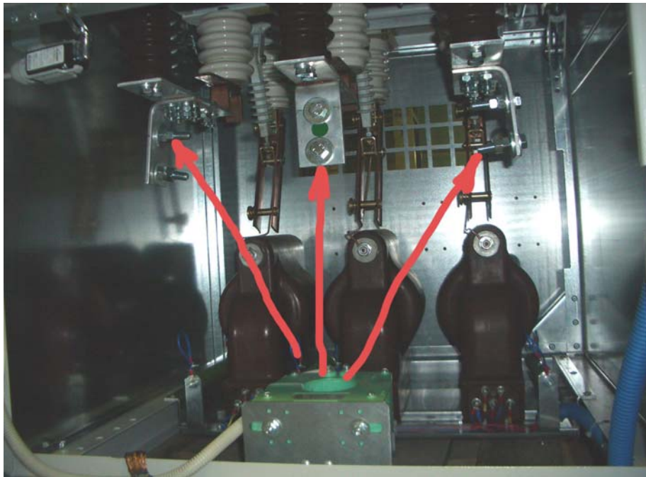
Камера КСО -207 ВВ монтаж кабеля в ячейке.
