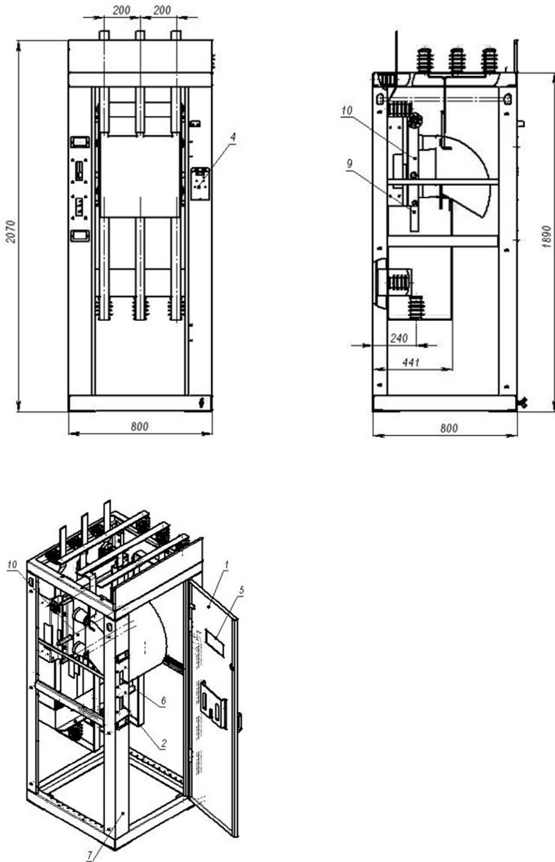
Рис. 2 Общий вид и габаритные размеры КСО-386М схемы 018
