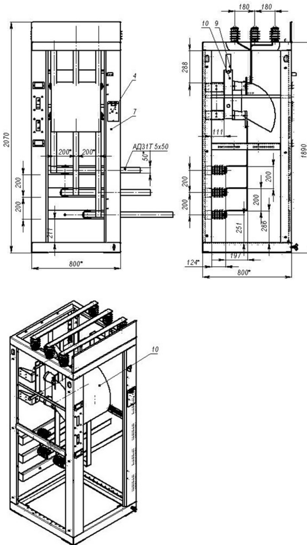
Рис. 3 Общий вид и габаритные размеры КСО-386М схемы 019
