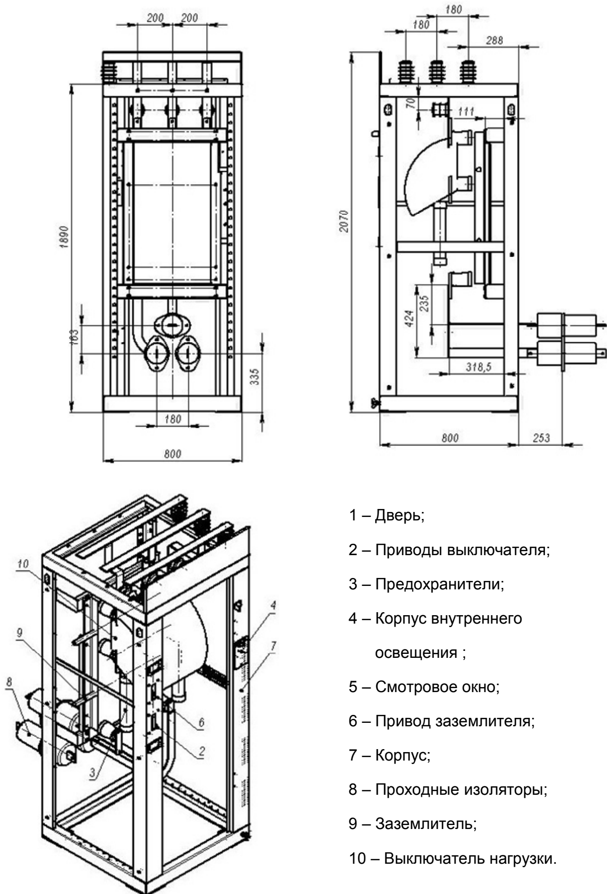
Рис. 1 Общий вид и габаритные размеры КСО-386М схемы 017
